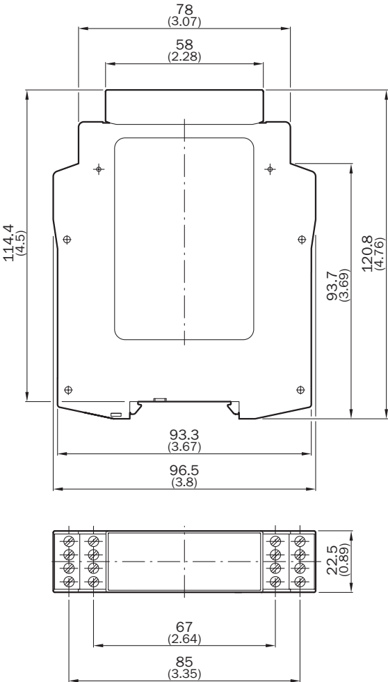
Esquema de dimensiones Módulo principal Flexi Classic
