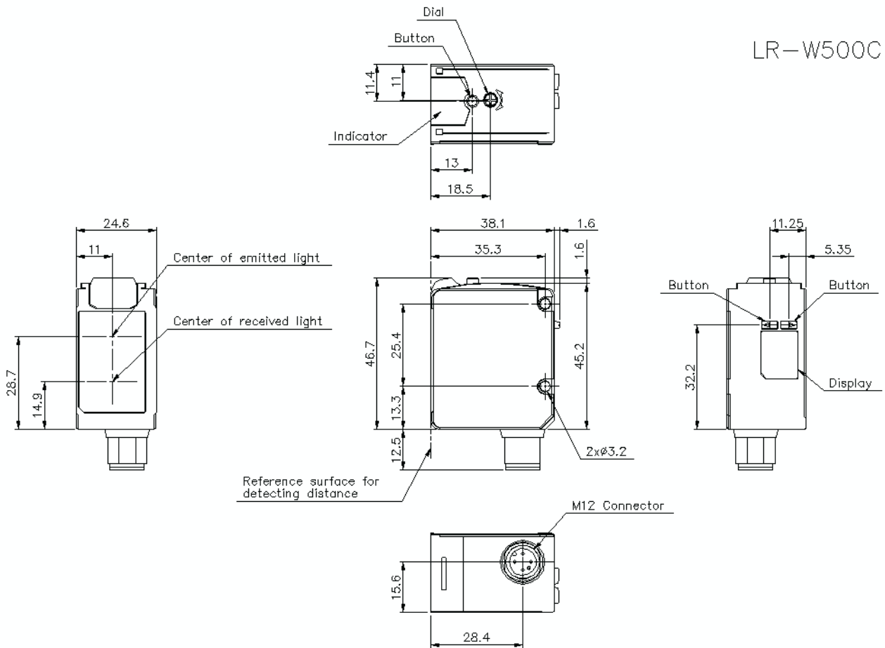
lr-w500c_dimension_01.gif
